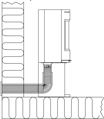
Kuva 2A, ulkoseinän läpi
