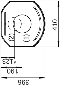
(1) - Center rökrör (2) - Center frisklufttillförsel
