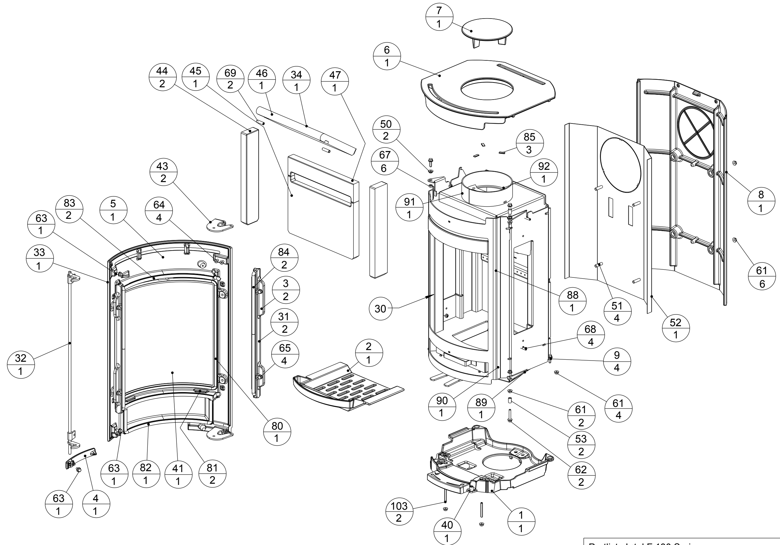
Partlist, Jøtul F 130 Serien
